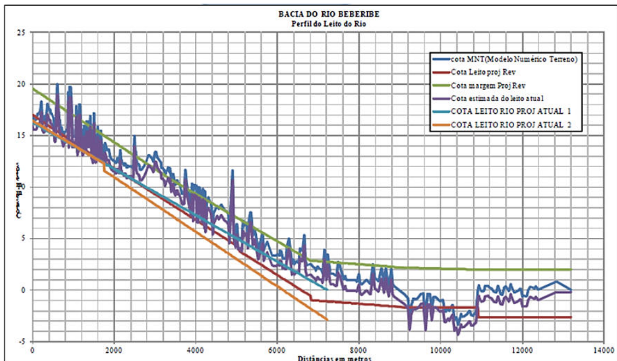
Figura 65: Perfil Projetado para o Beberibe
