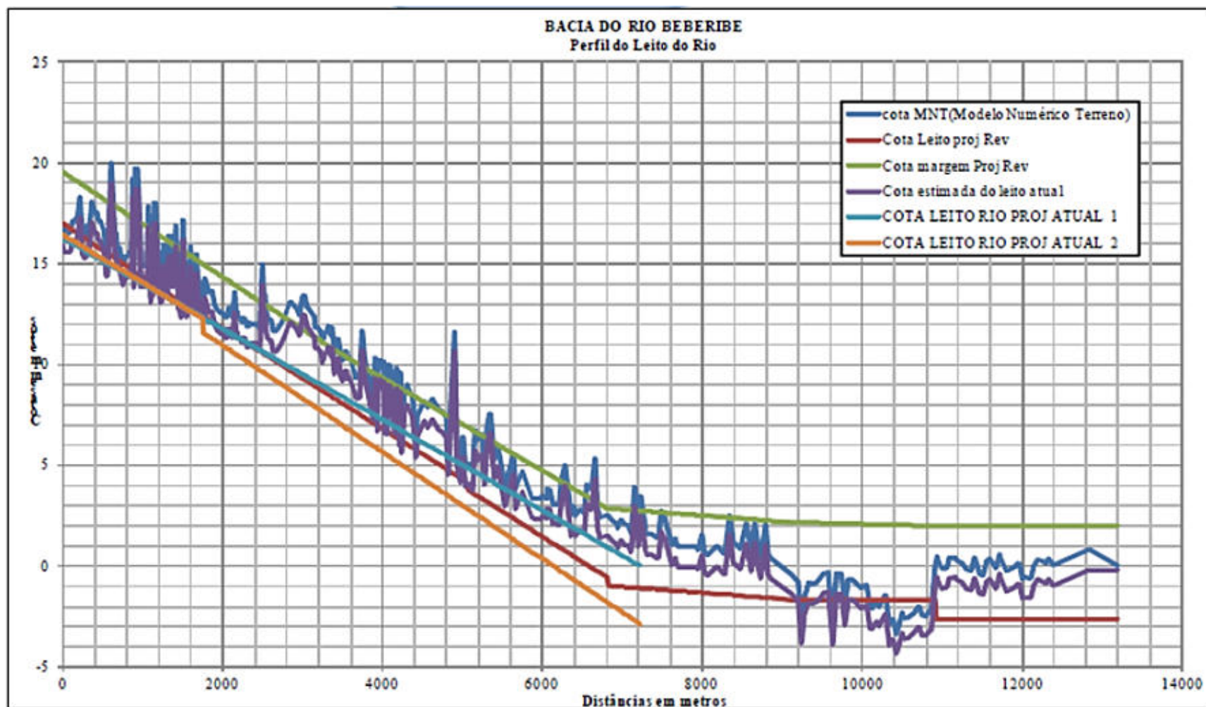
Figura 98: Gráfico Perfis Longitudinais Propostos para o Rio Beberibe
