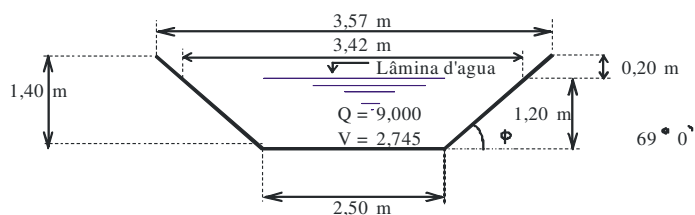
Figura 75: Dados da Seção do Canal do Buriti
