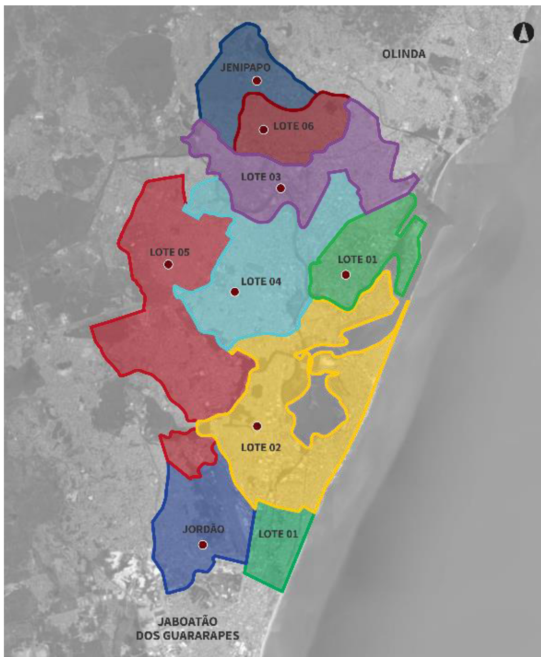
Figura 29: PROMAIS - Projeto de Setorização de Rede e Implantação dos Distritos de Medição e Controle: Planície do Recife.
