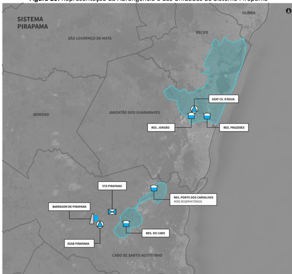
Figura 20: Representação da Abrangência e das Unidades do Sistema Pirapama
