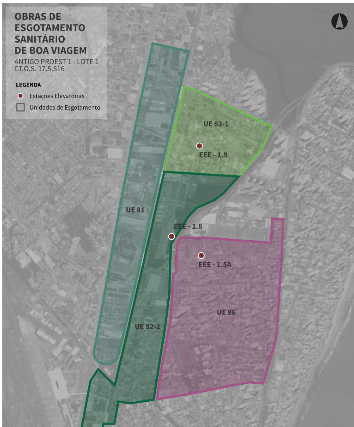
Figura 49: Área de Abrangência do Sistema de Esgotamento Sanitário de Boa Viagem
