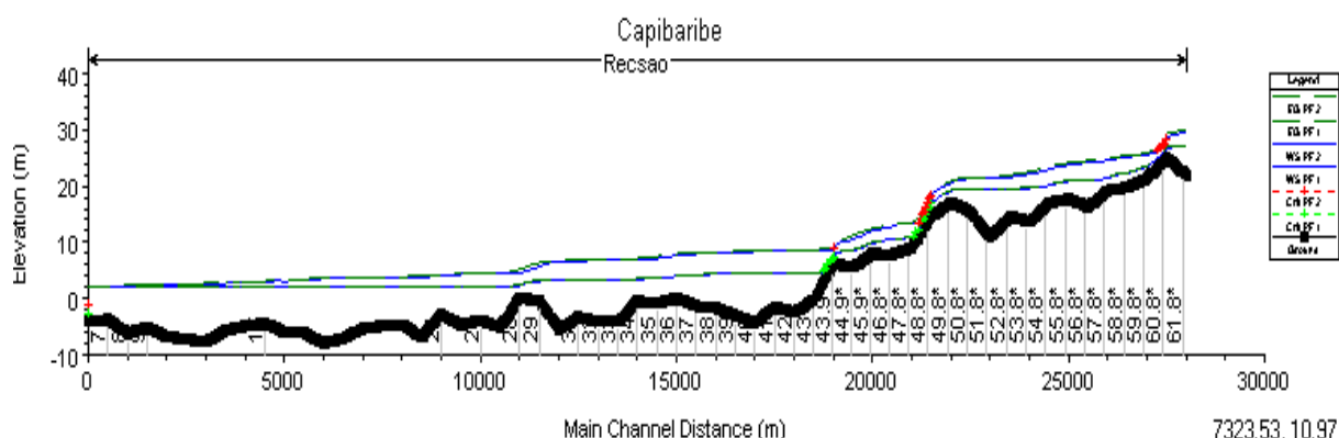
Figura 64: Hidrograma de Cheia para TR=10 ANOS – Capibaribe
