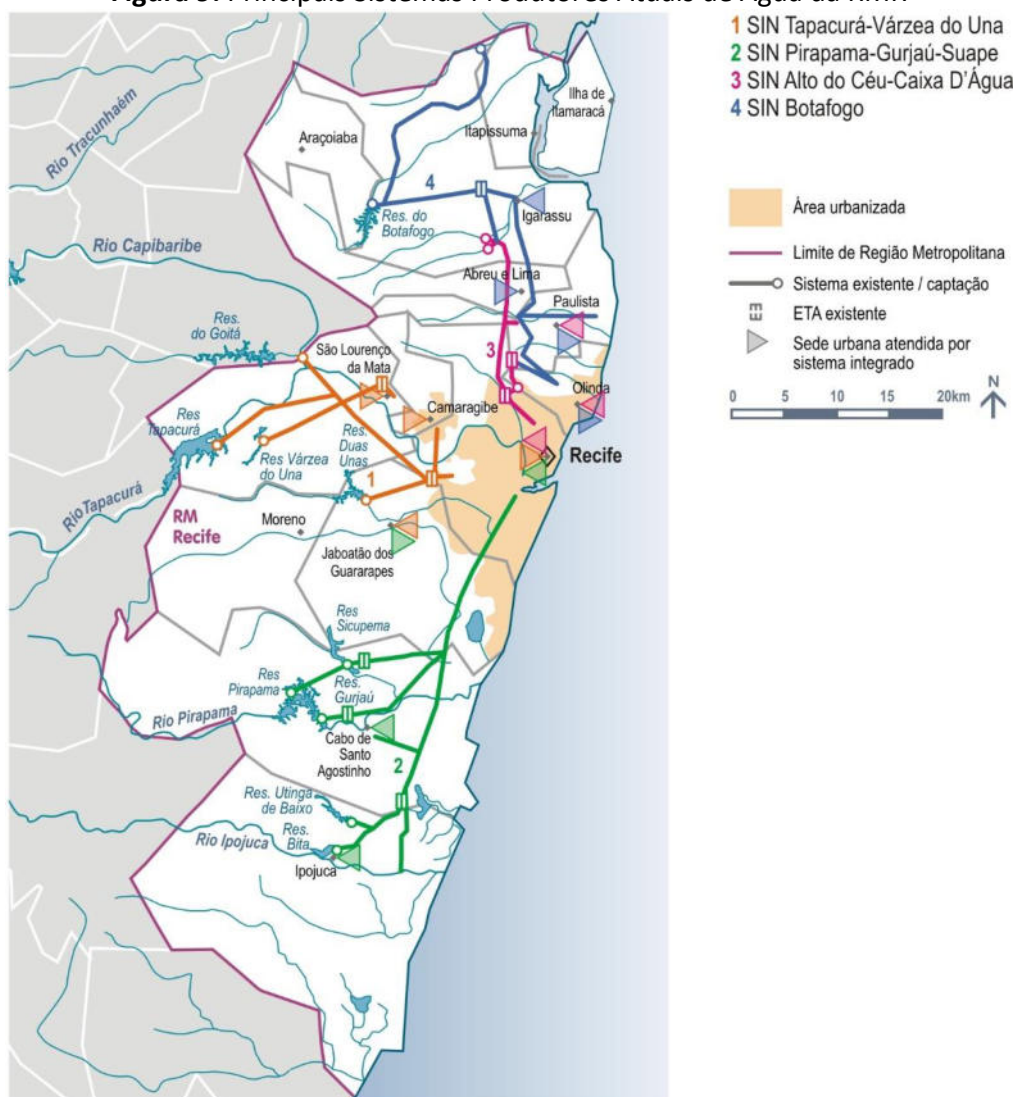
Figura 9: Principais Sistemas Produtores Atuais de Água da RMR
