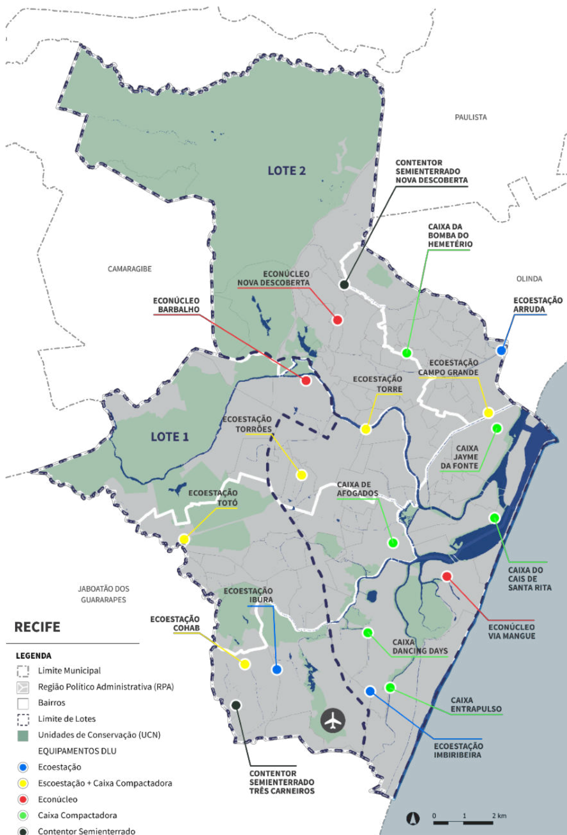
Figura 134: Mapa da Localização das Ecoestações, Econúcleos, Caixas Compactadoras e Contentores nos Lotes 01 e 02.
