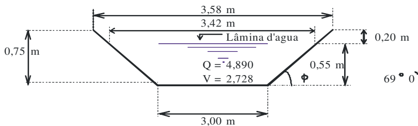
Figura 79 - Dados do Trecho 1 - Canal do Parnamirim
