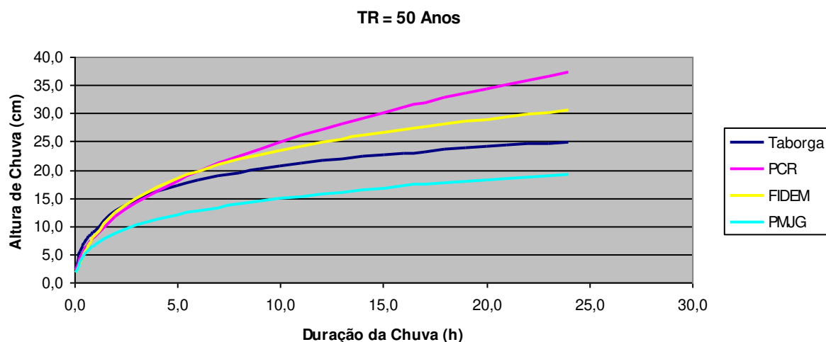
Figura 59: Alturas de Chuvas para T = 50 anos.
