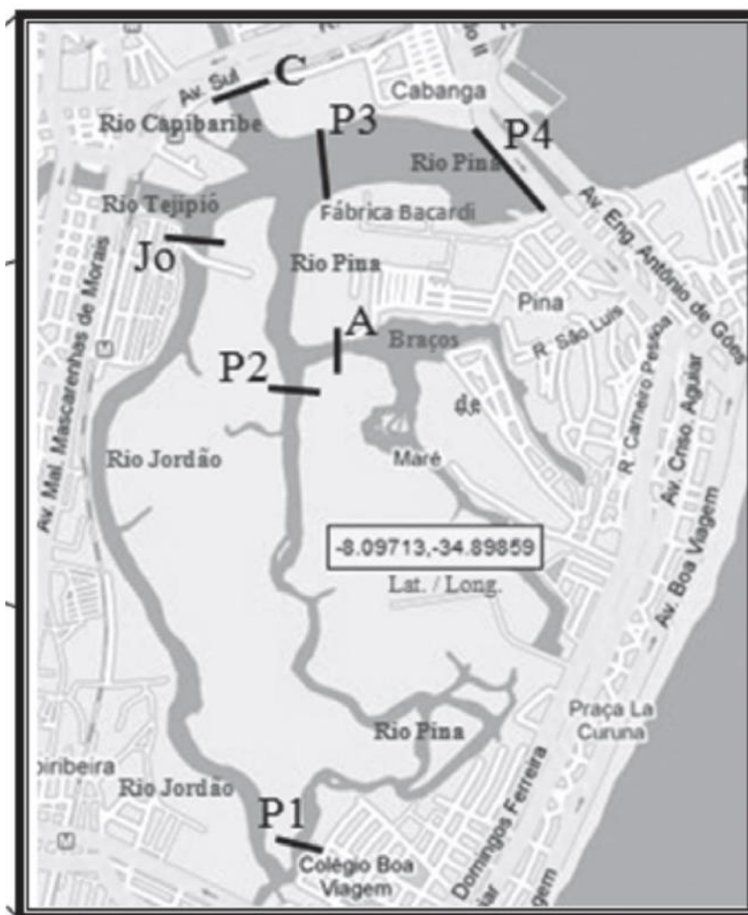
Figura 63: Localização dos Pontos Onde Foram Realizadas as Medições linimétricas
