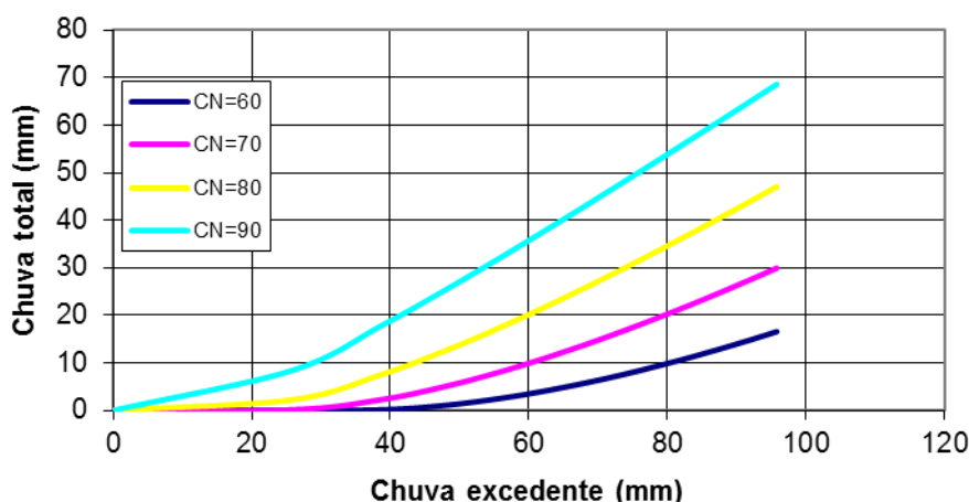
Figura 60: Chuva Excedente para Vários Valores de CN
