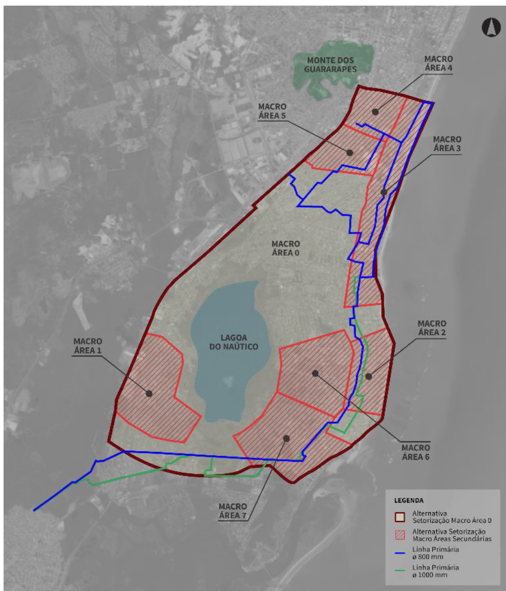
Figura 31: PROMAIS - Projeto de Setorização de Rede e Implantação dos Distritos de Medição e Controle: Jaboatão dos Guararapes.
