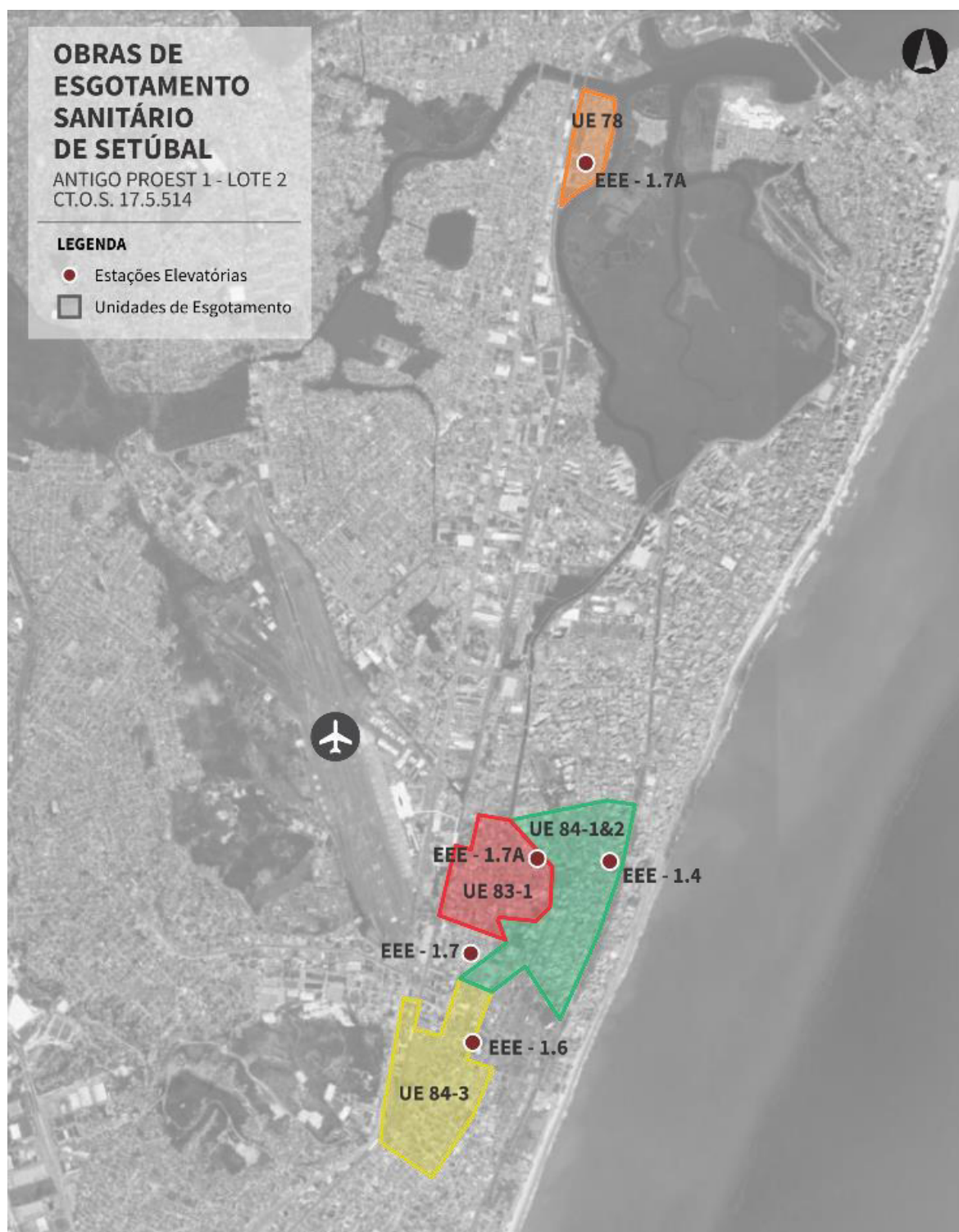
Figura 50: Área de Abrangência do Sistema de Esgotamento Sanitário de Setúbal
