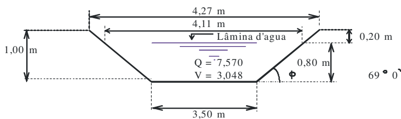
Figura 81: Dados do Trecho 3 – Canal do Parnamirim
