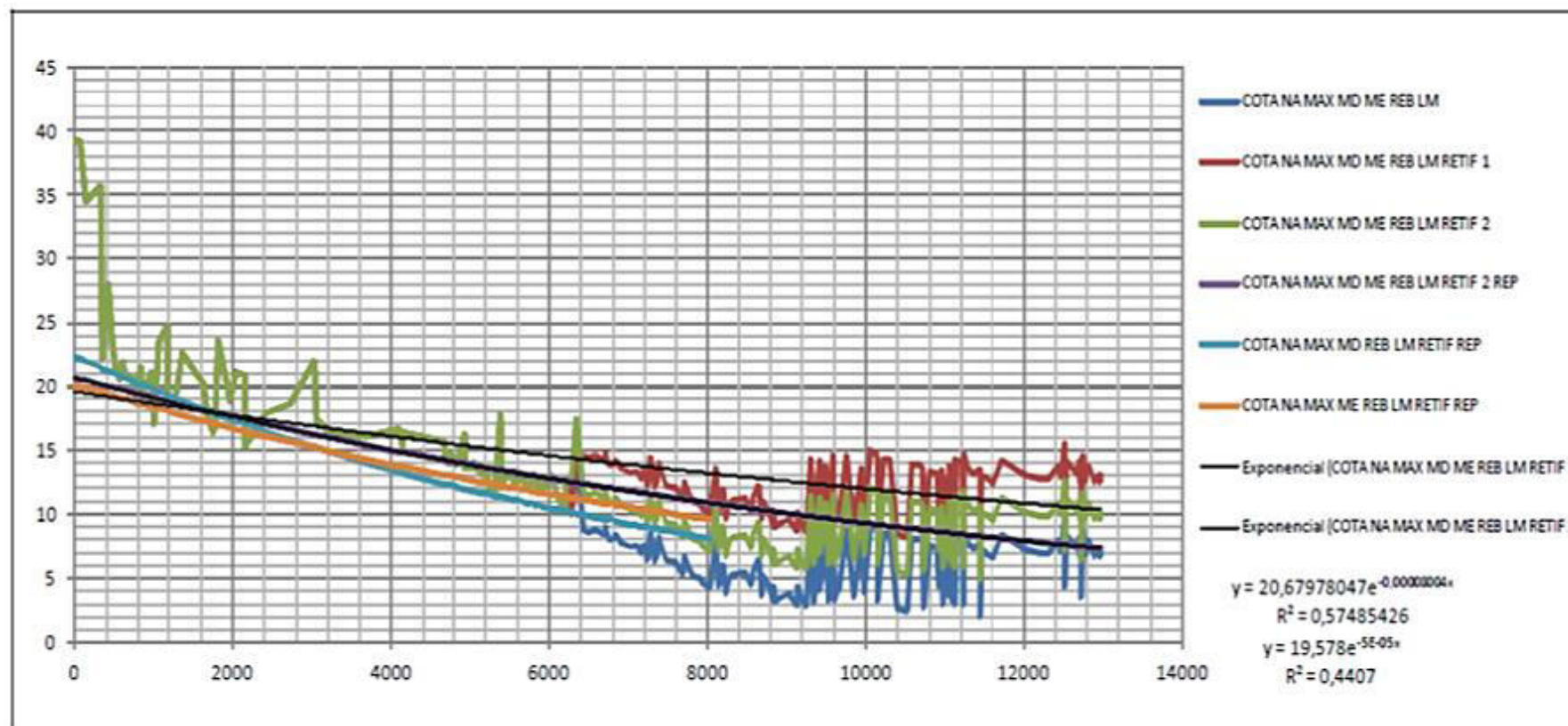
Figura 97: Gráfico da Cota Média da Envoltória de Cheia na Calha do Beberibe.
