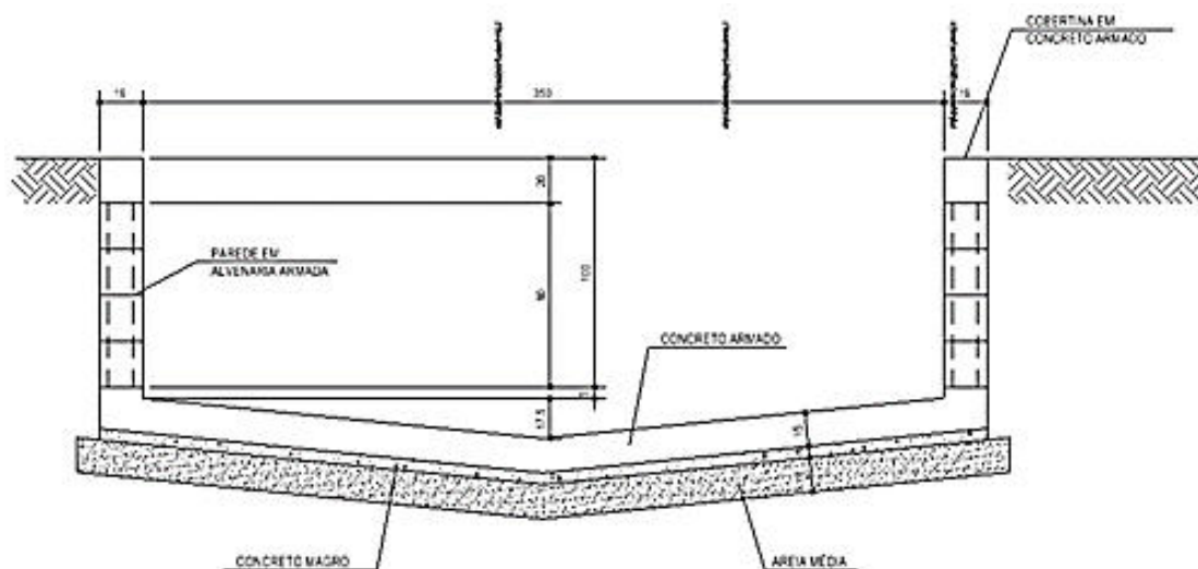
Figura 90: Seção Tipo Projetada para o Canal.
