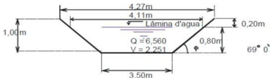
Figura 80 - Dados do Trecho 2 - Canal do Parnamirim.
