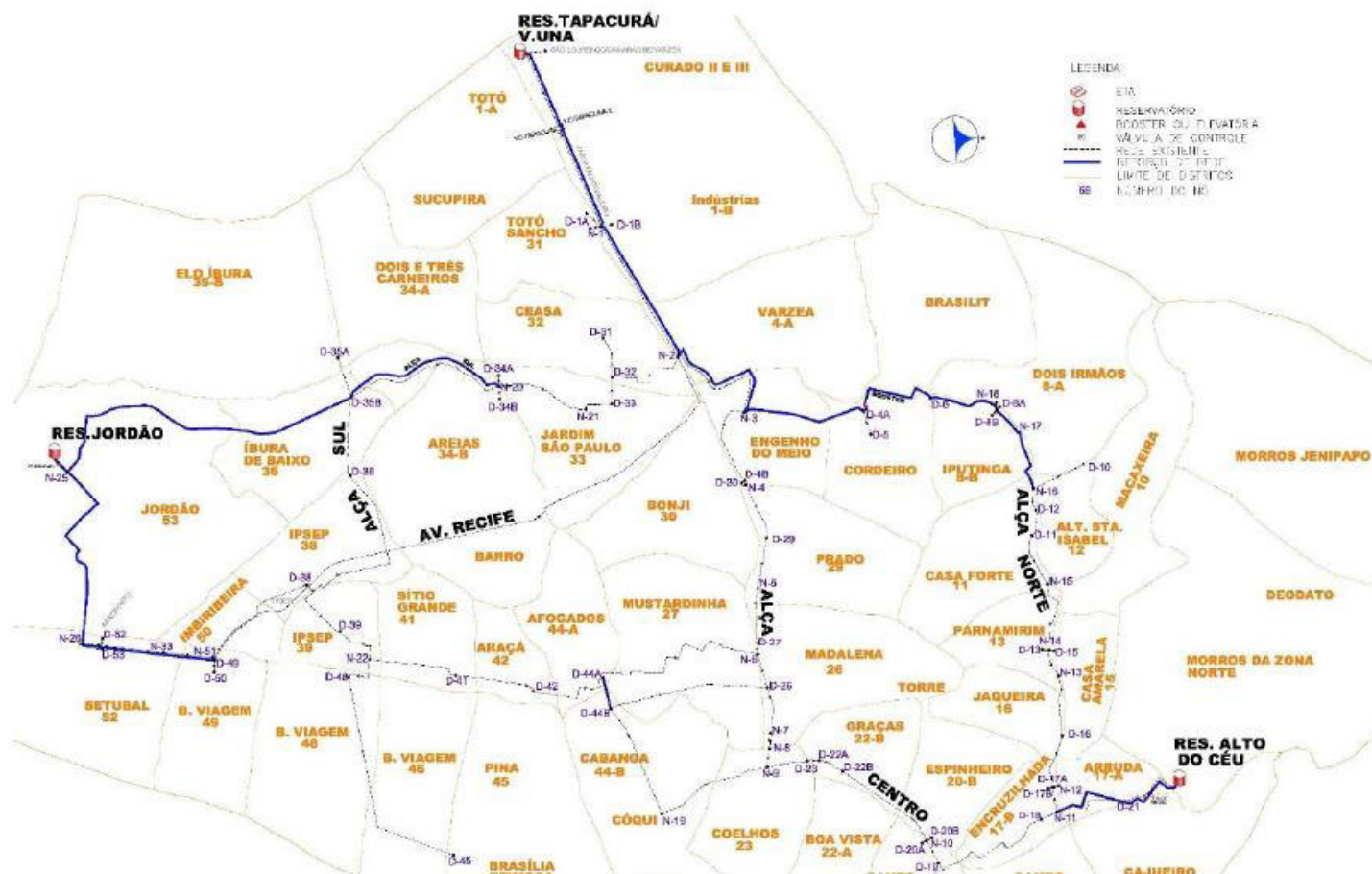
Figura 16: Interdependência Hidráulica e Funcional dos Grandes Anéis de Distribuição da Rede do Recife e Seus Distritos e/ou Setores de Medição e Controle – SMC ou DMC.
