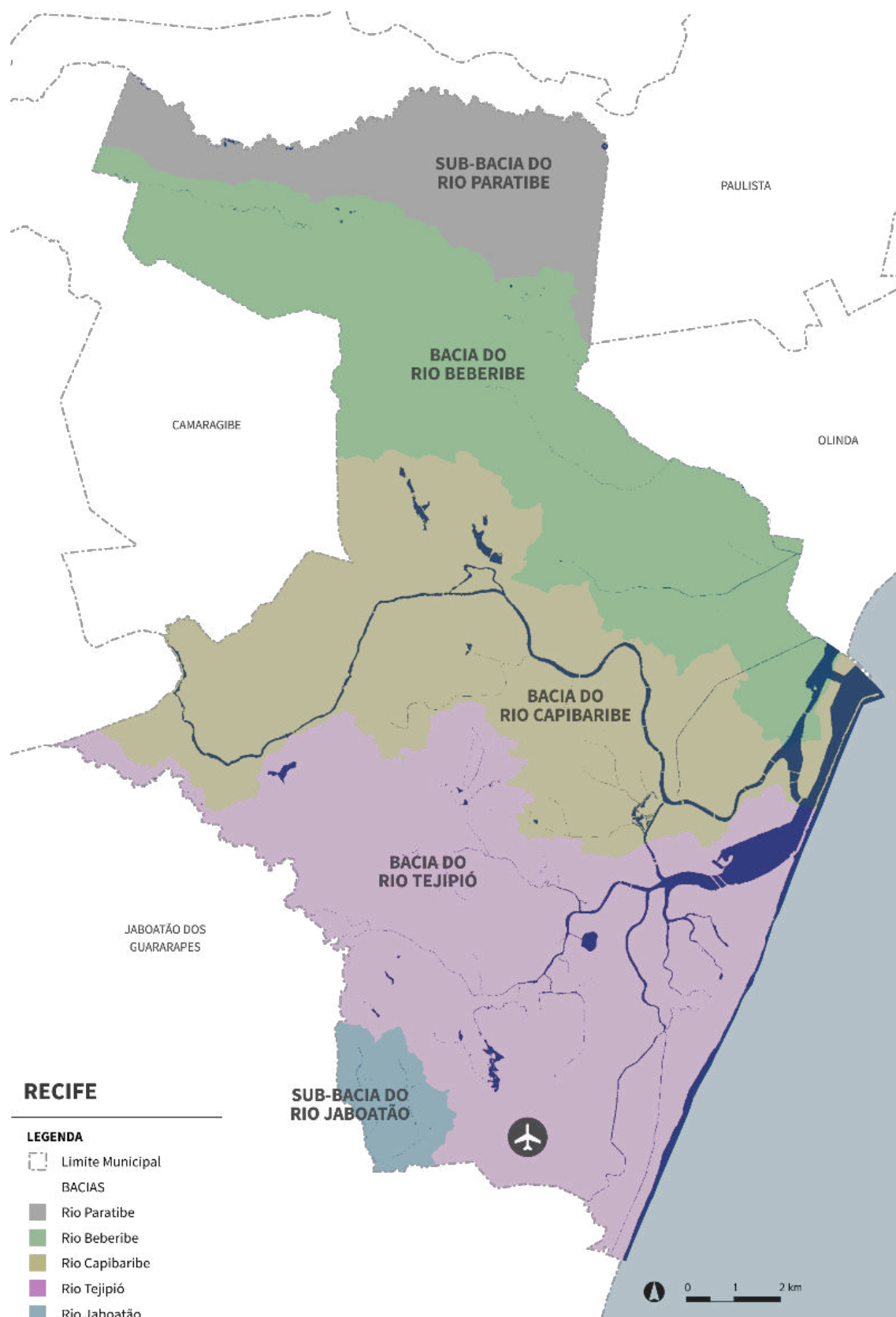
Figura 55: Bacias Hidrográficas do Recife.
